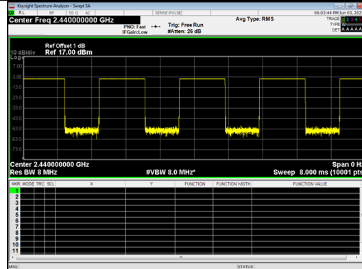
BLE 2M_Channel 19
