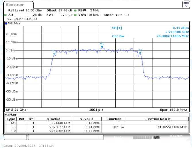
11AX80MIMO-Ant2-5210
