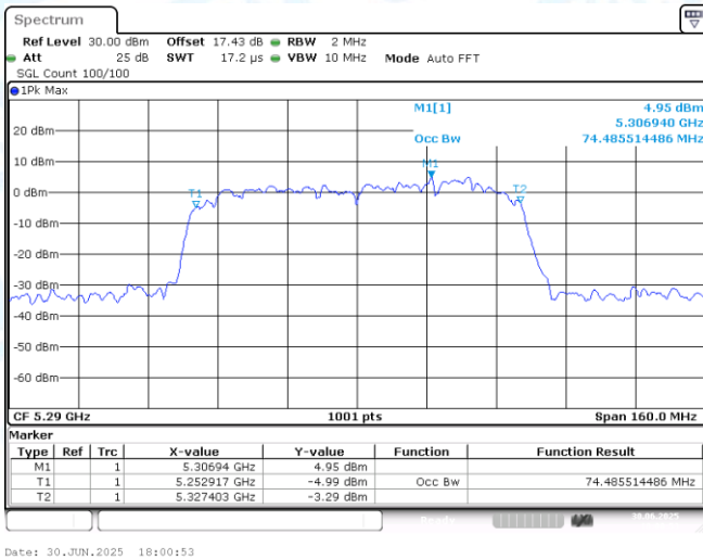
11AX80MIMO-Ant1-5290
