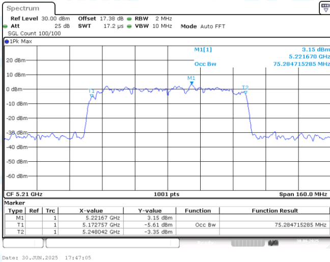
11AX80MIMO-Ant1-5210
