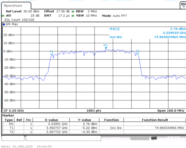
11AX80MIMO-Ant1-5530
