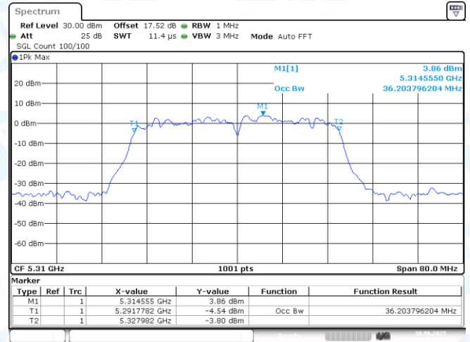
11AX40MIMO-Ant2-5310
