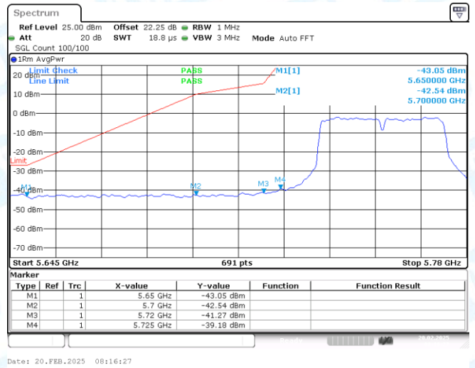
11N40SISO-Ant1-5755-PASS
