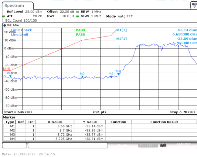
11N40SISO-Ant1-5755-PASS
