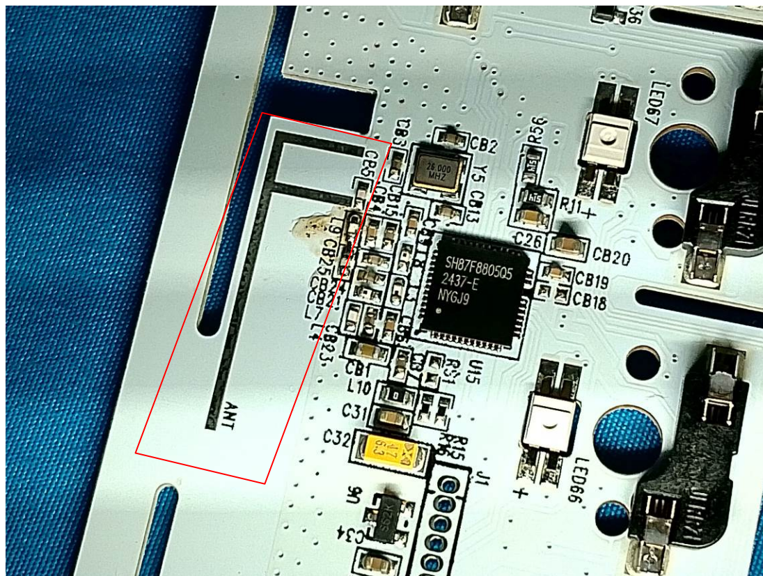
BLE&SRD Antenna
