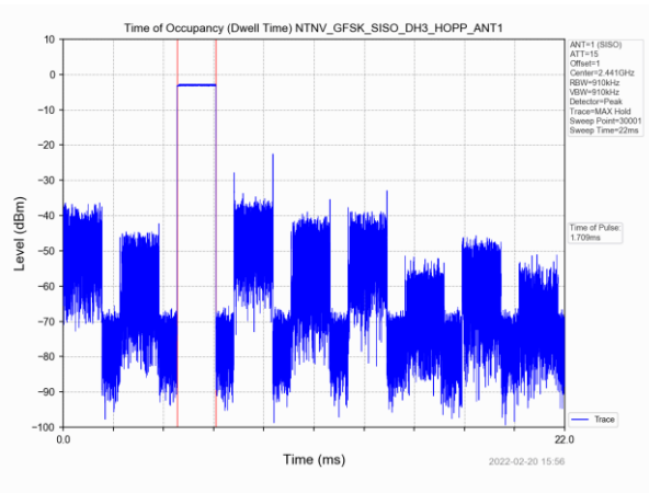
DH3
