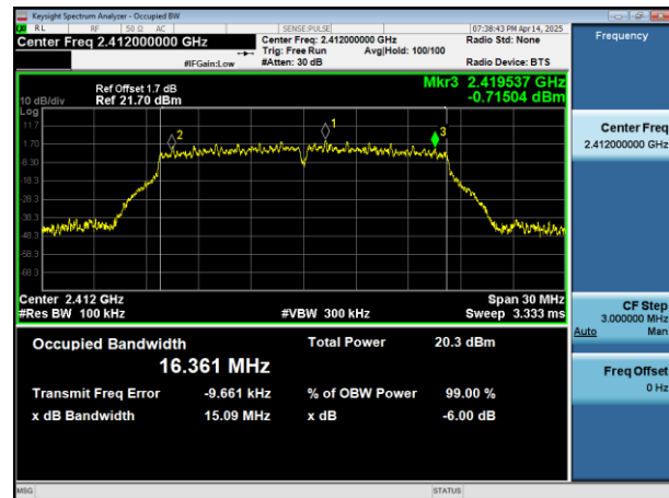
802.11g_ANT 2
