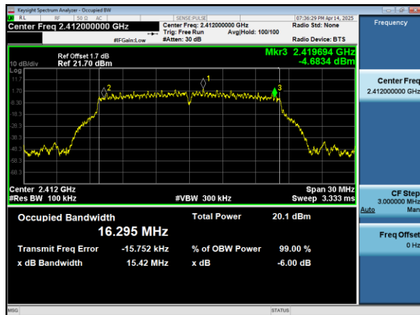
802.11g_ANT 1
