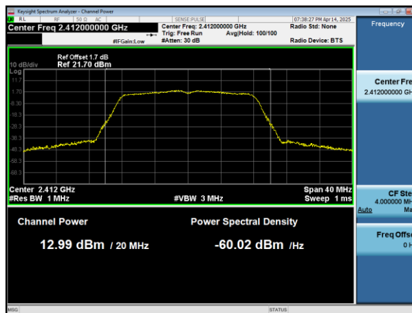
802.11g_ANT 2
