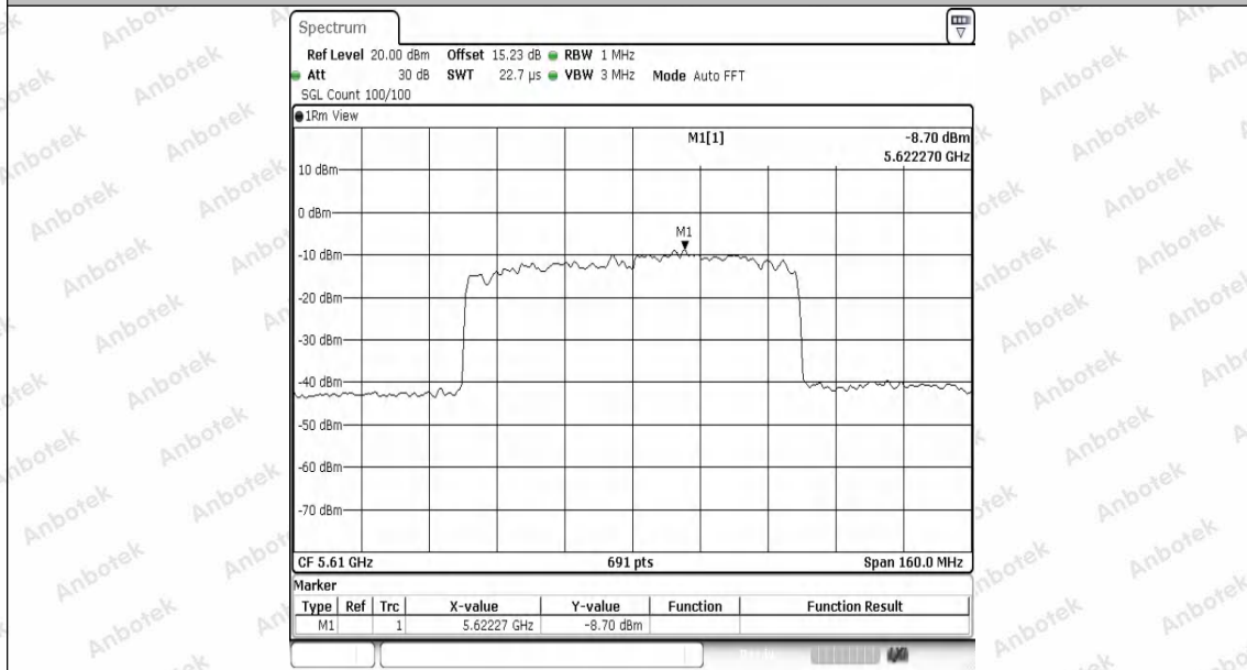
11AX80SISO-Ant1-5610-PASS
