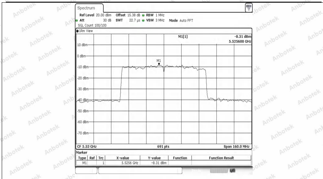
11AC80SISO-Ant1-5530-PASS
