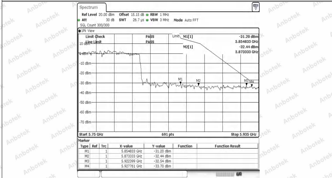
11AC80SISO-Ant1-5775-PASS
