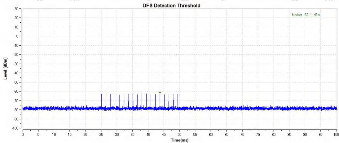
11AX80SISO_5530_Type0
