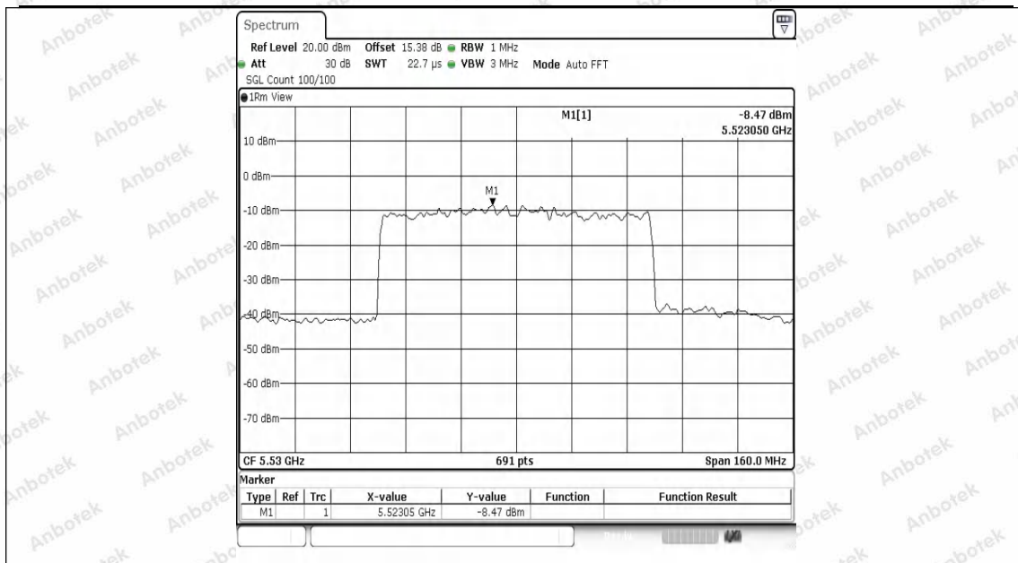
11AX80SISO-Ant1-5530-PASS
