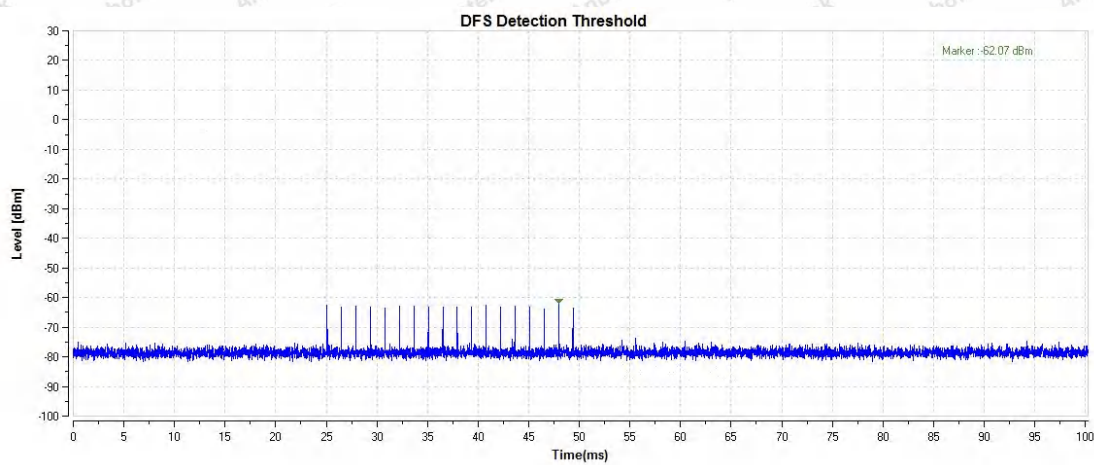
11AX80SISO_5530_Type0
