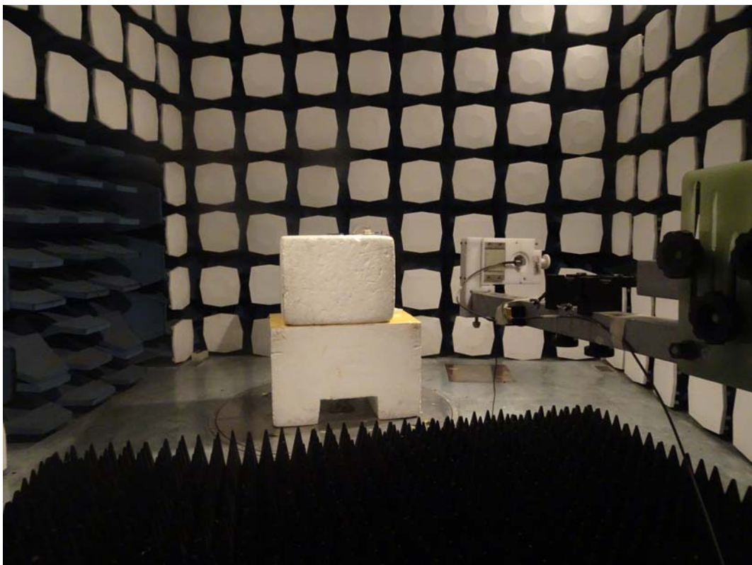
18GHz-26.5GHz
