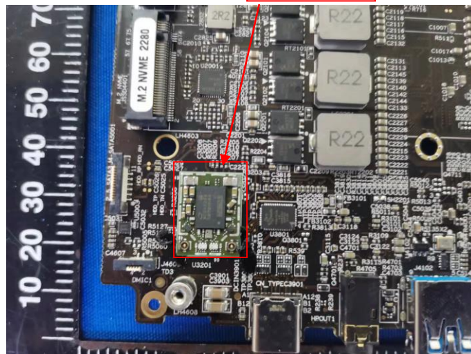
RF Module
