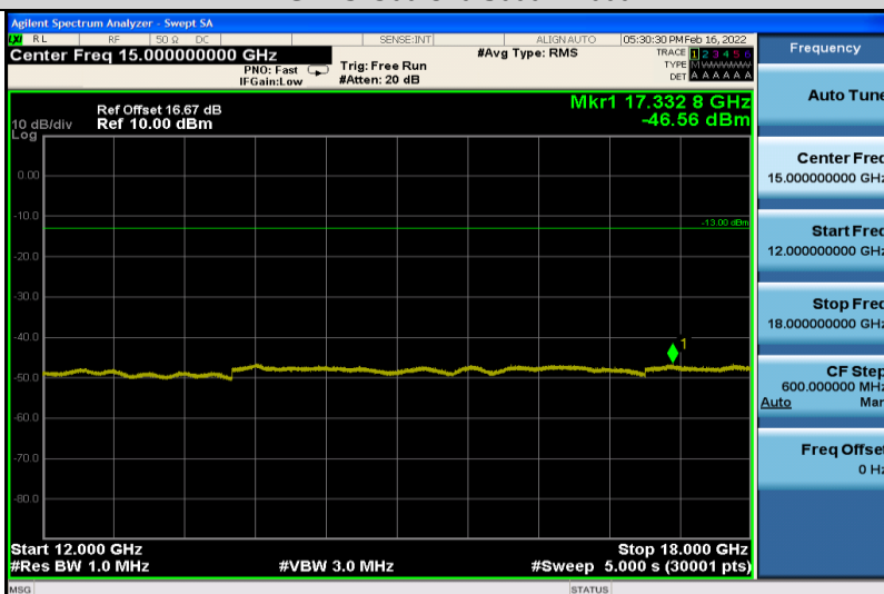
EGPRS1900-810-12000~18000
