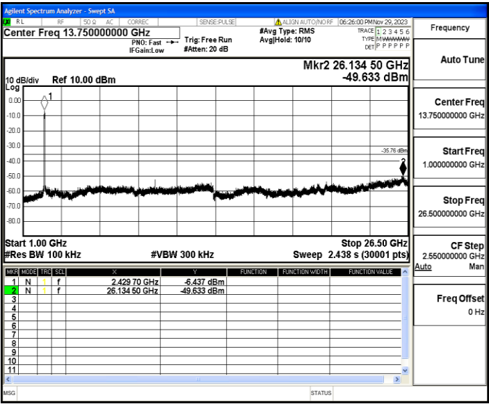
11N40MIMO_Ant2_2437_0~Reference
