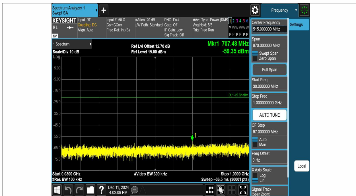
2.4G DTS-Ant1-2480-30~1000-PASS
