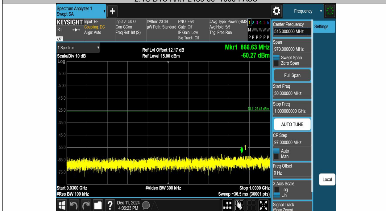
2.4G DTS-Ant2-2480-30~1000-PASS
