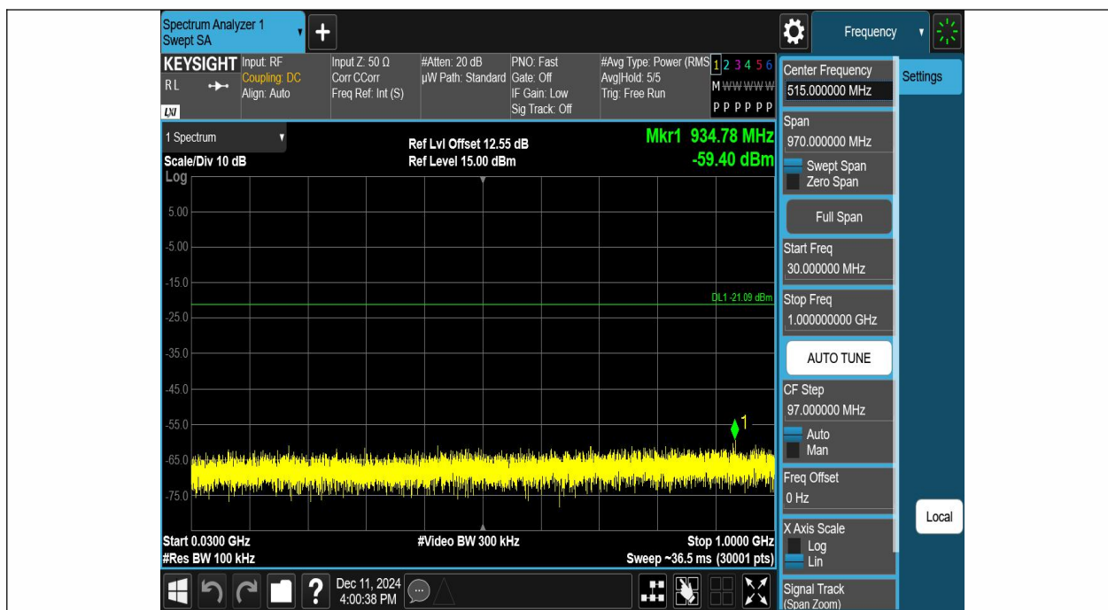
2.4G DTS-Ant1-2440-30~1000-PASS
