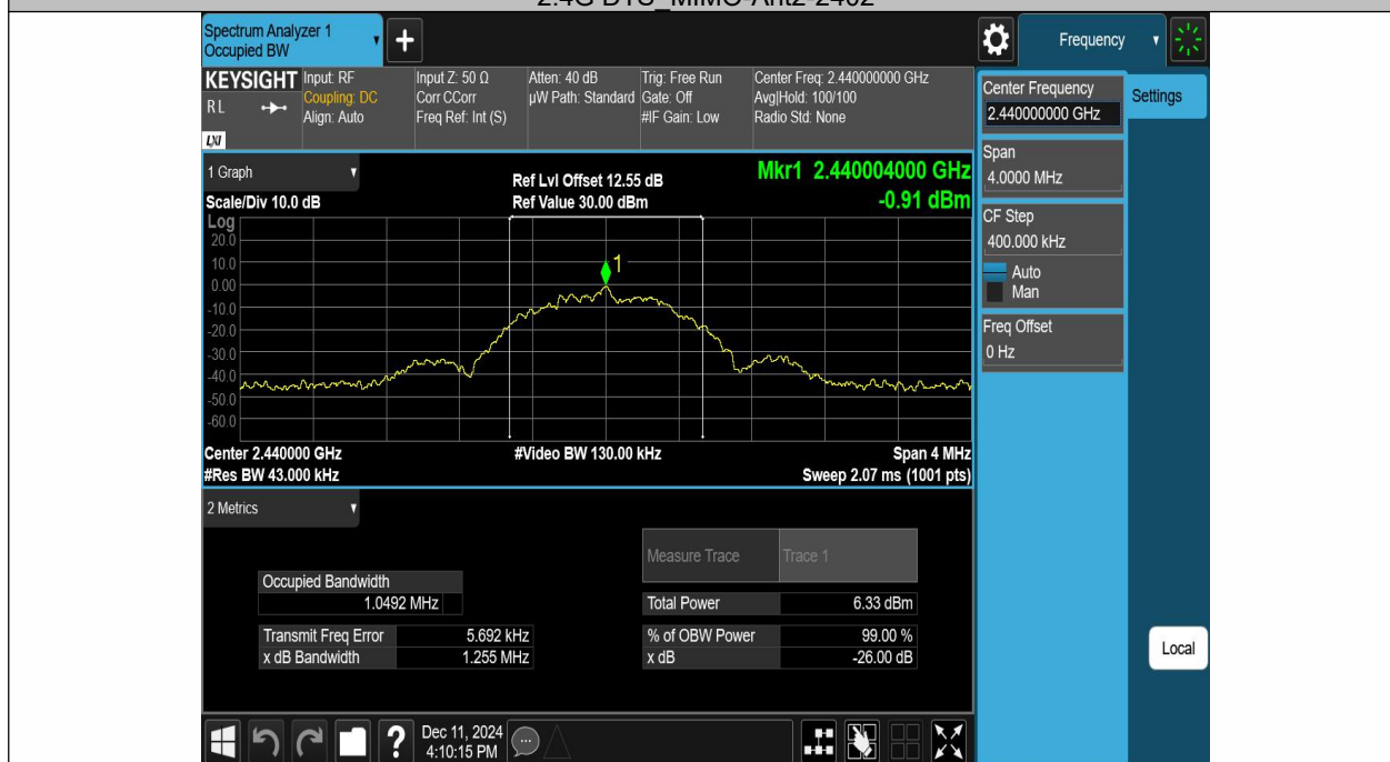
2.4G DTS MIMO-Ant1-2440
