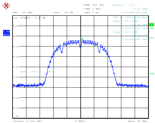
b_2412MHz_Chain 0 15.720MHz
