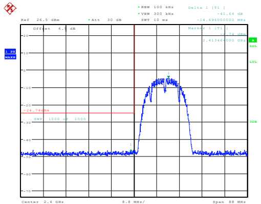
b_2412MHz_Chain 0 41.64dB
