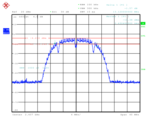
b_2437MHz_Chain 0 13.120MHz
