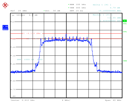
n20_2412MHz_Chain 0 15.160MHz
