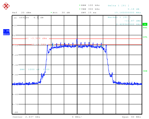
n20_2437MHz_Chain 0 15.160MHz
