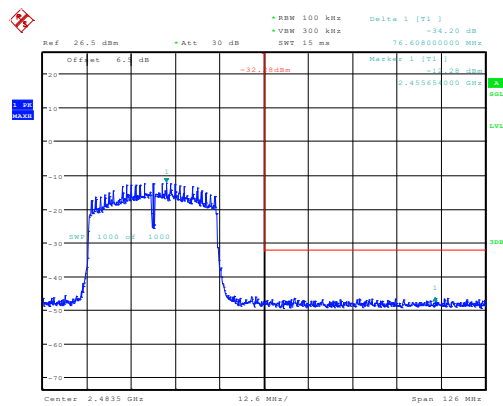
n40_2452MHz_Chain 0 34.20dB
