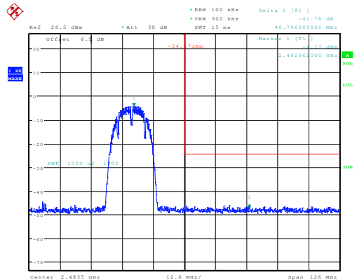
b_2462MHz_Chain 0 41.78dB
