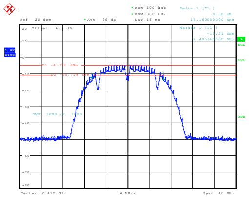
b_2412MHz_Chain 0 13.160MHz
