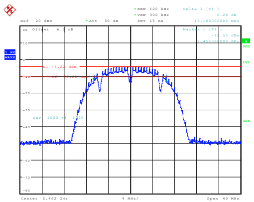
b_2462MHz_Chain 0 13.160MHz
