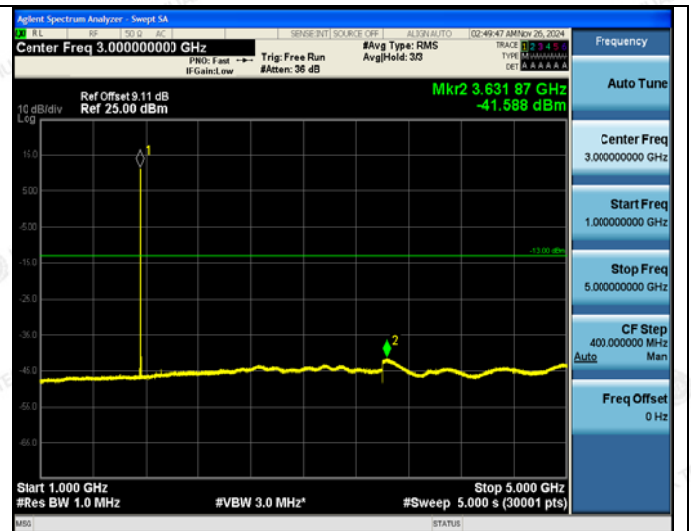
1GHz~5GHz
