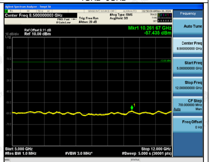
5GHz~12GHz
