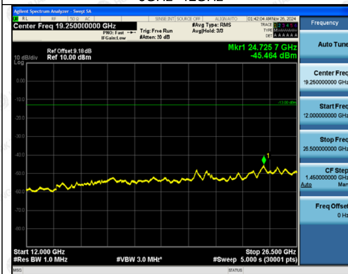
12GHz~26.5GHz
