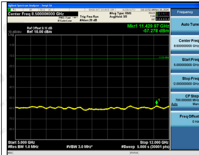
5GHz~12GHz
