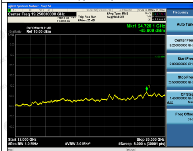
12GHz~26.5GHz
