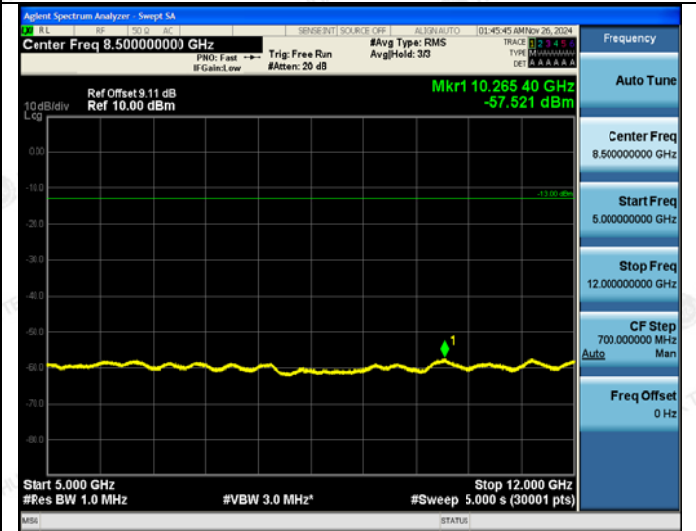
5GHz~12GHz
