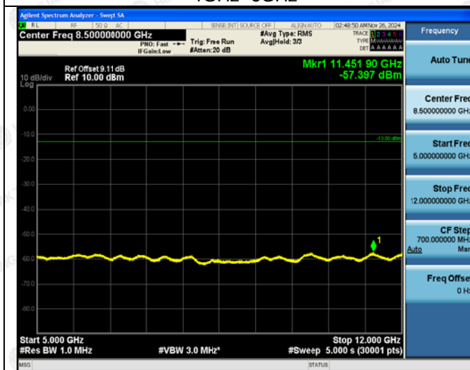
5GHz~12GHz
