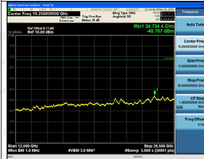
12GHz~26.5GHz
