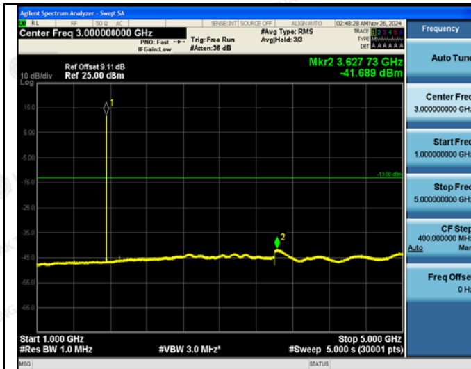
1GHz~5GHz
