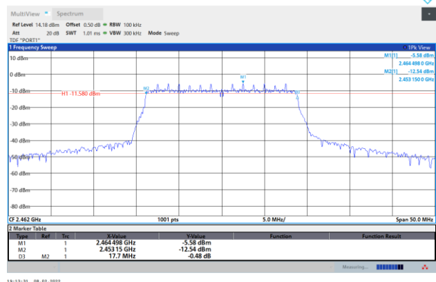
802.11n_HT20 / 2 462 MHz
