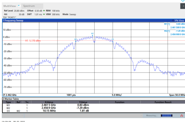
802.11b / 2 462 MHz
