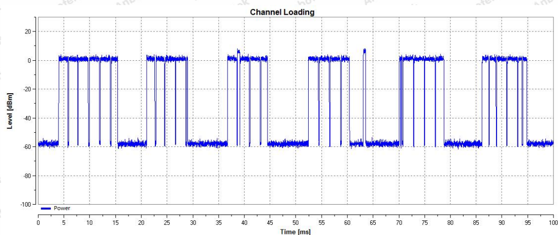
11AC80SISO_5610_Type0
