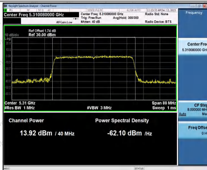
11AX40SISO_Ant2_5310
