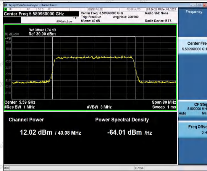
11AX40SISO_Ant2_5590
