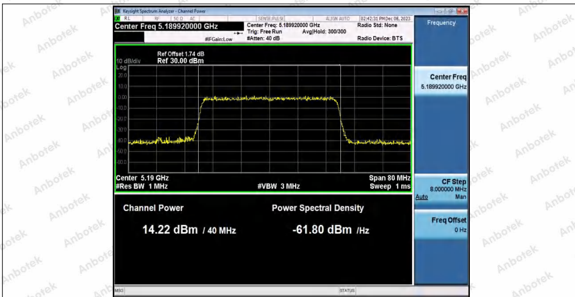
11AX40SISO_Ant2_5190
