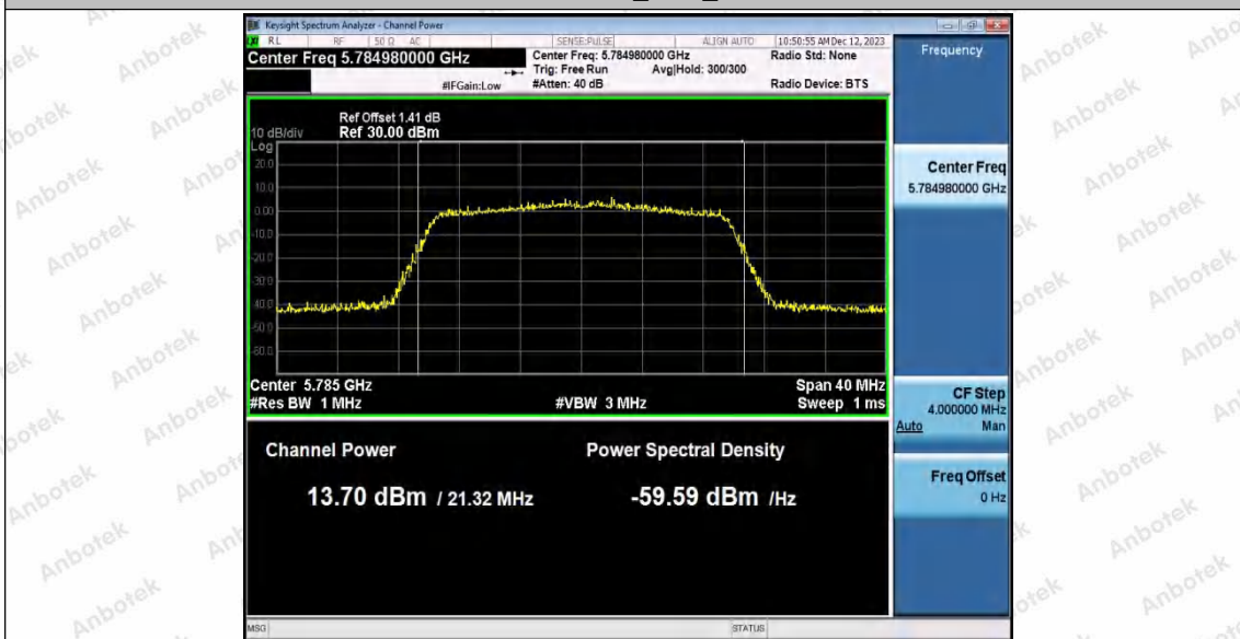
11AX20SISO_Ant2_5785
