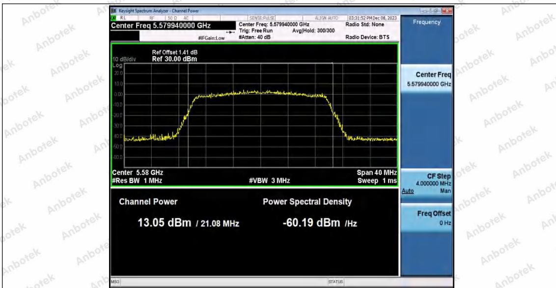
11AX20SISO_Ant2_5580
