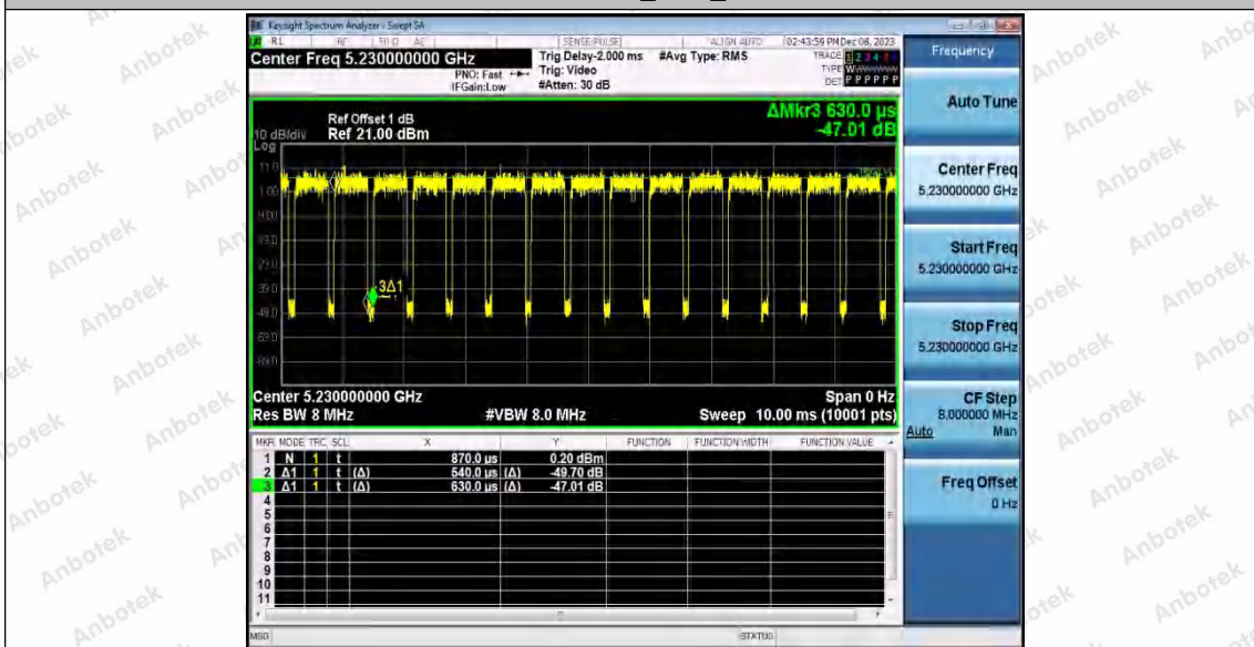
11AX40SISO_Ant1_5230
