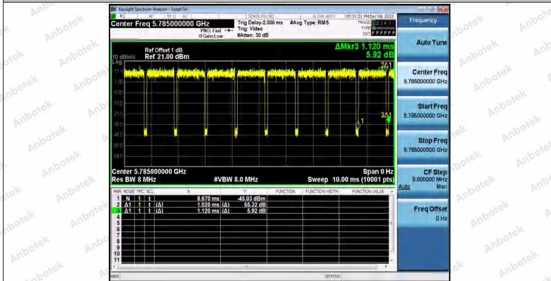
11AX20SISO_Ant2_5785
