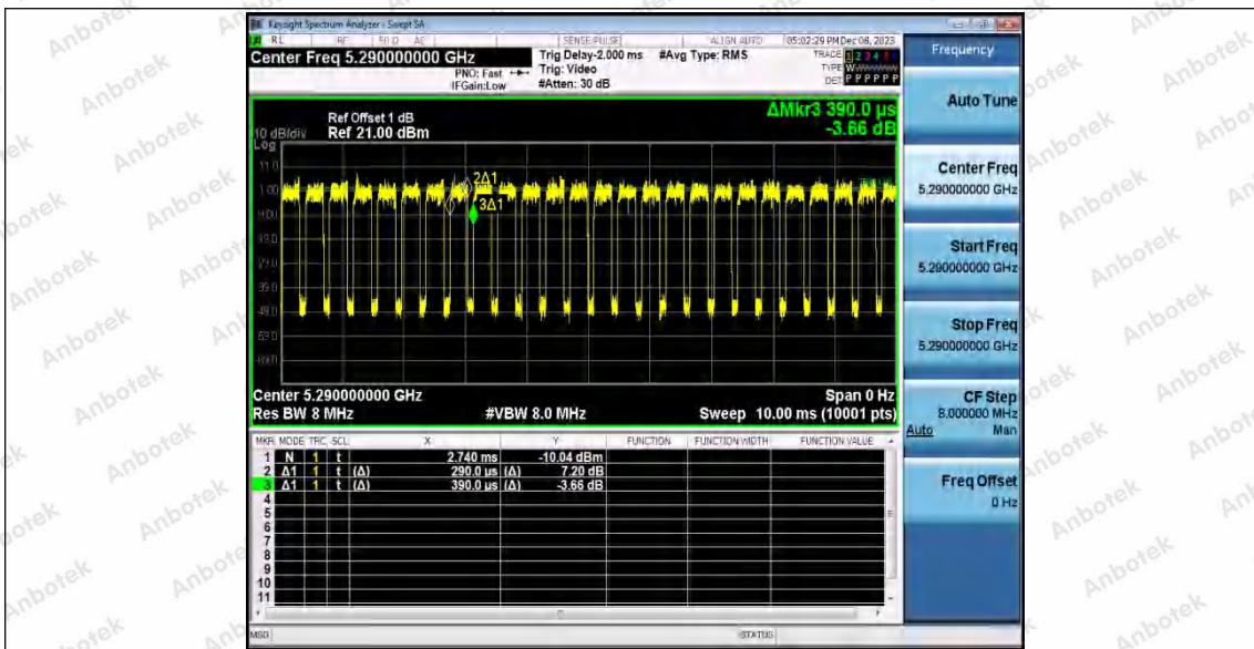
11AX80SISO_Ant2_5290
