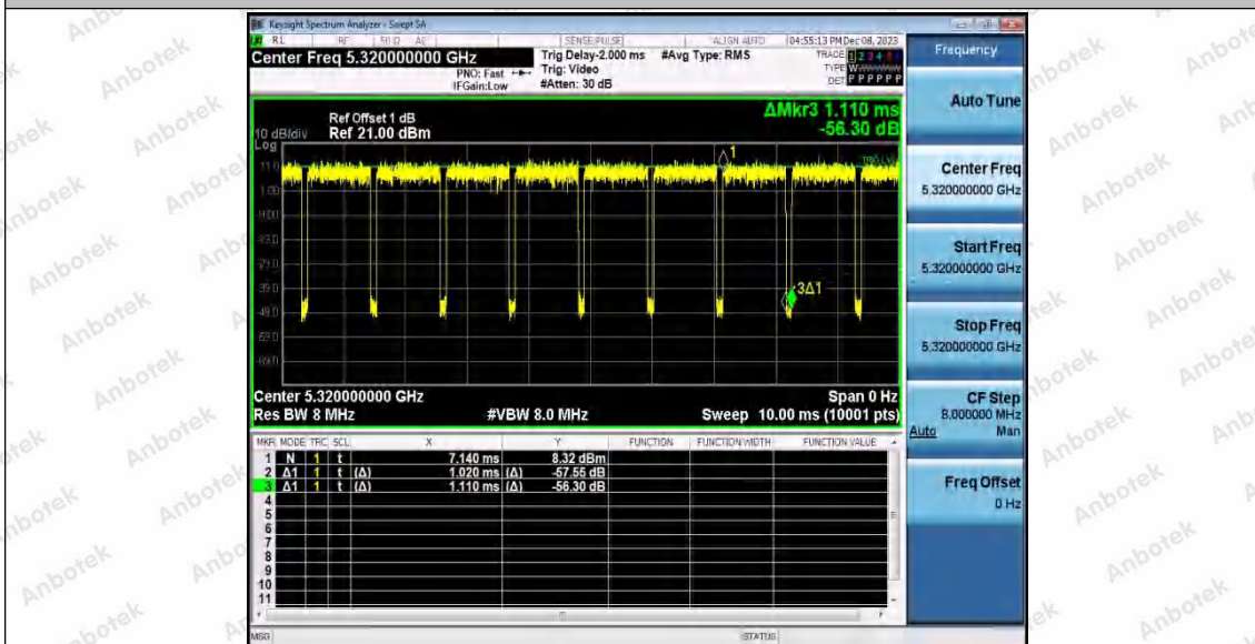
11AX20SISO_Ant2_5320
