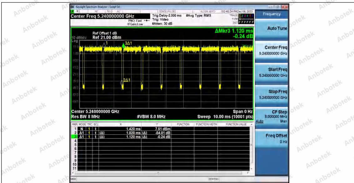
11AX20SISO_Ant2_5240
