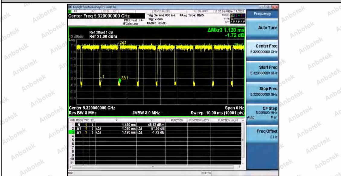
11AX20SISO_Ant2_5320
