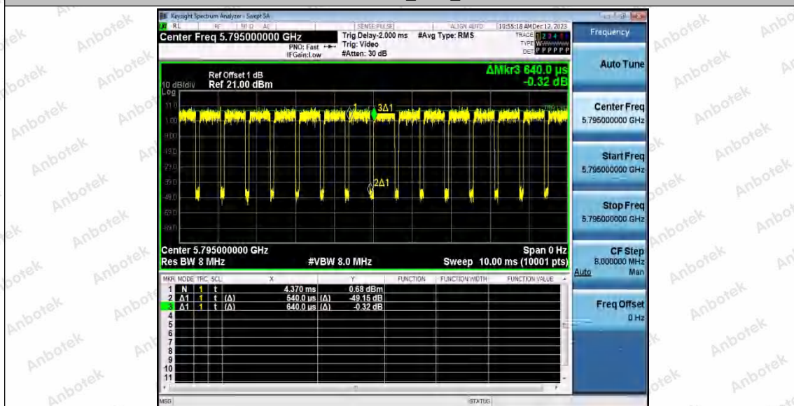
11AX40SISO_Ant2_5795
