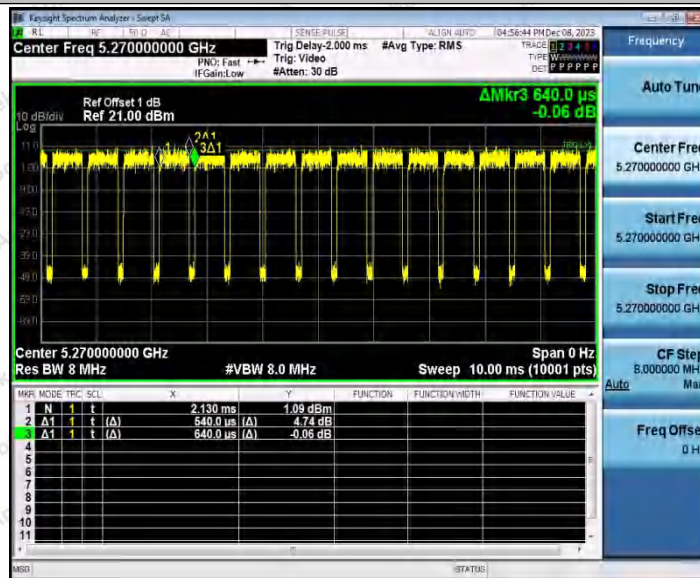
11AX40SISO_Ant2_5270
