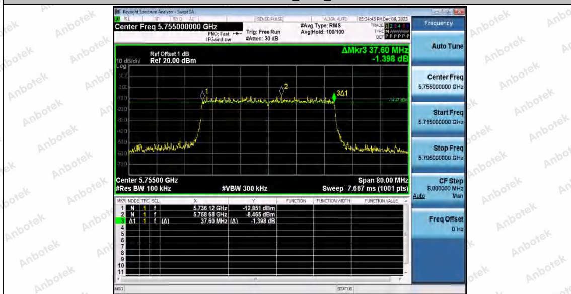
11AX40ISO_Ant1_5755
