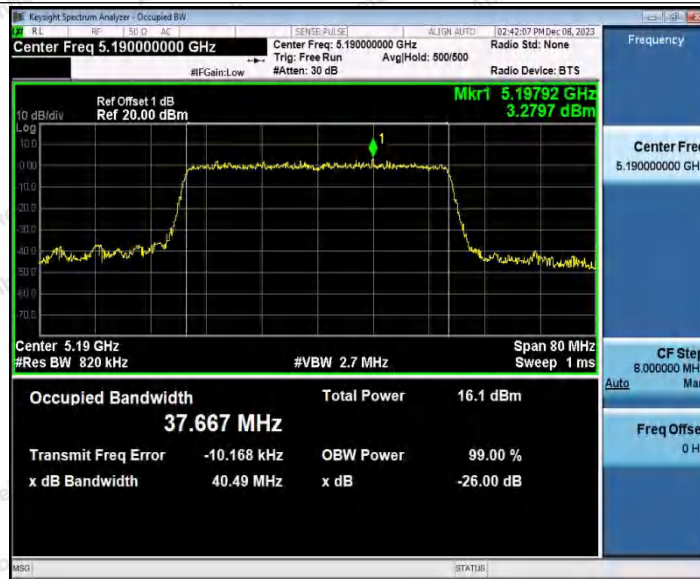
11AX40SISO_Ant2_5190
