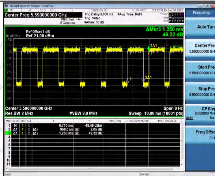
11N40SISO_Ant2_5590
