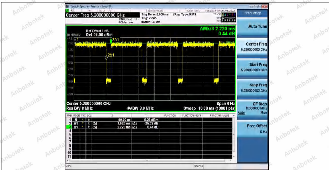
11N20SISO_Ant2_5280
