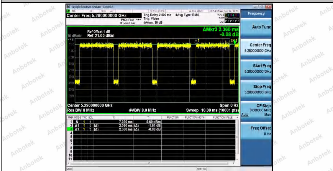
11A_Ant2_5280
