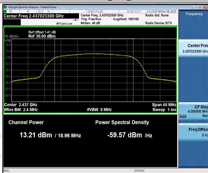
11AX20SISO_Ant2_2437
