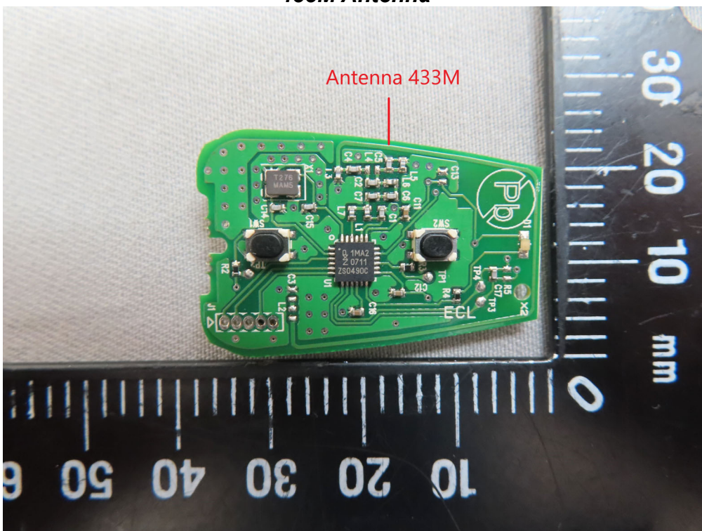
433M Antenna
