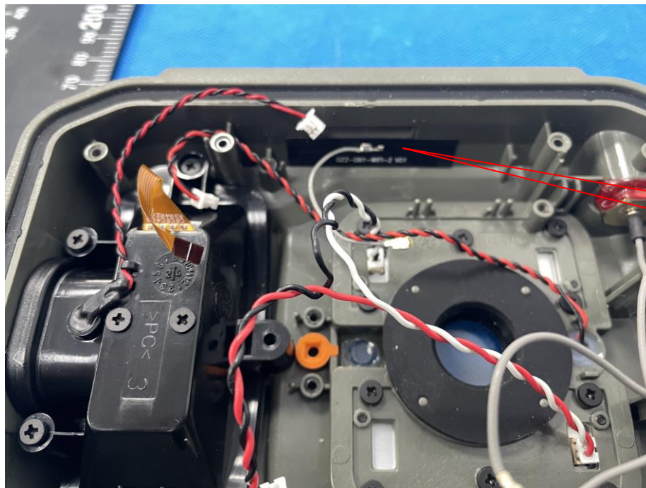
BT/WIFI Antenna
