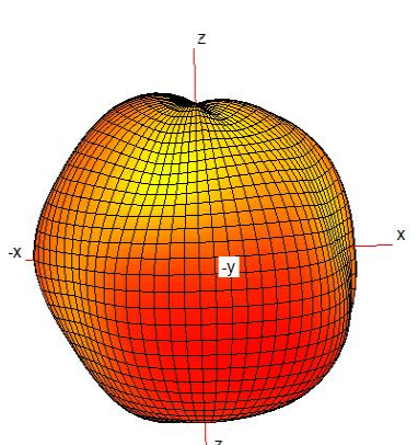
1700MHz
