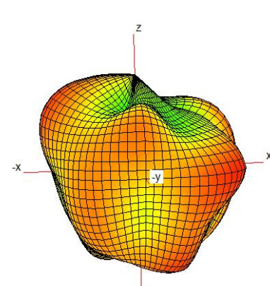
2100MHz
