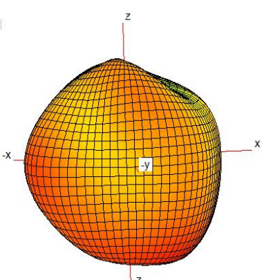
2000MHz
