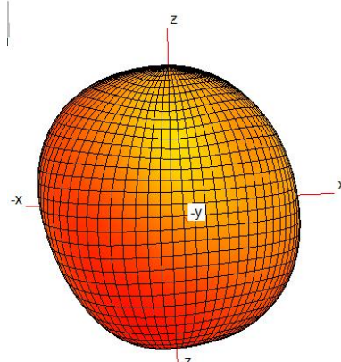
1900MHz
