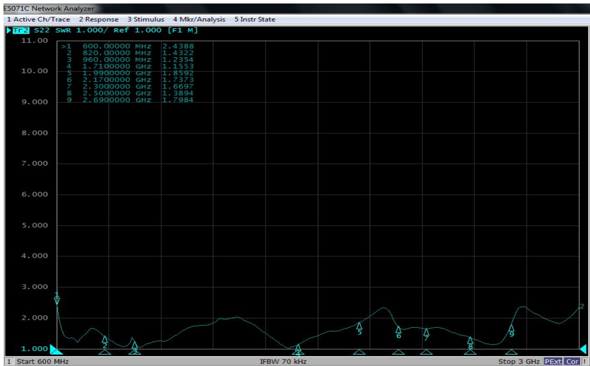
600~2700MHz antenna VSWR
