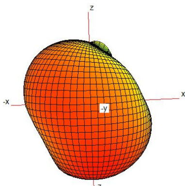
700MHz
