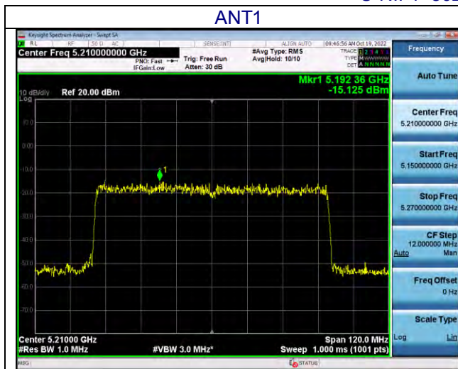
CH42 5210MHz
