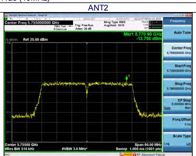
CH151 -5755MHz
