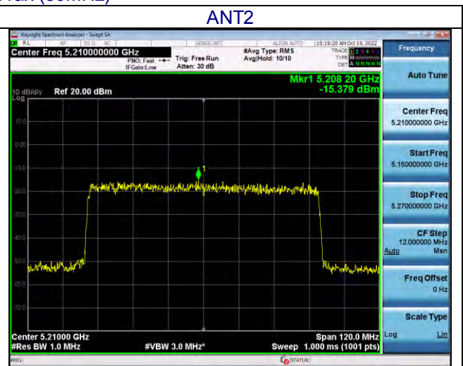
CH42 5210MHz
