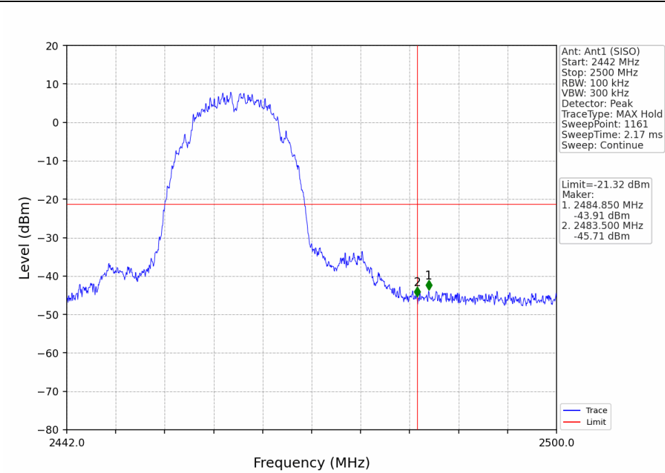
802.11b_HCH_2462MHz_Ant1 (SISO)_NTNV
