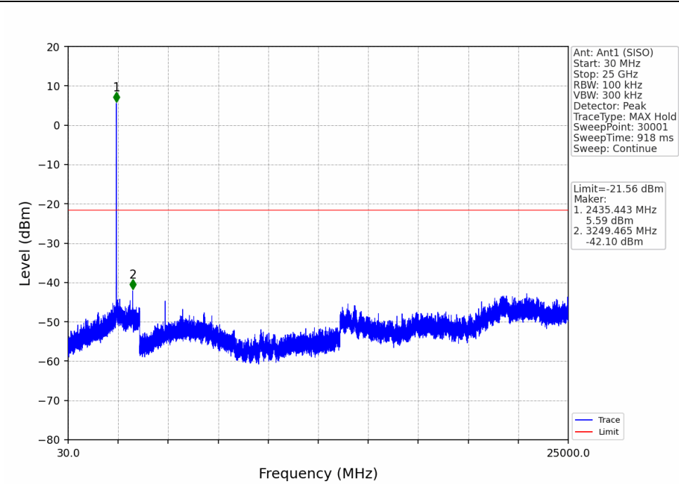
802.11b_MCH_2437MHz_Ant1 (SISO)_NTNV
