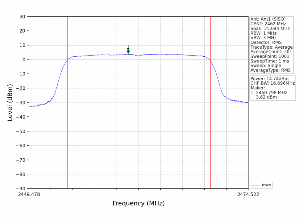
802.11g_HCH_2462MHz_Ant1 (SISO)_NTNV
