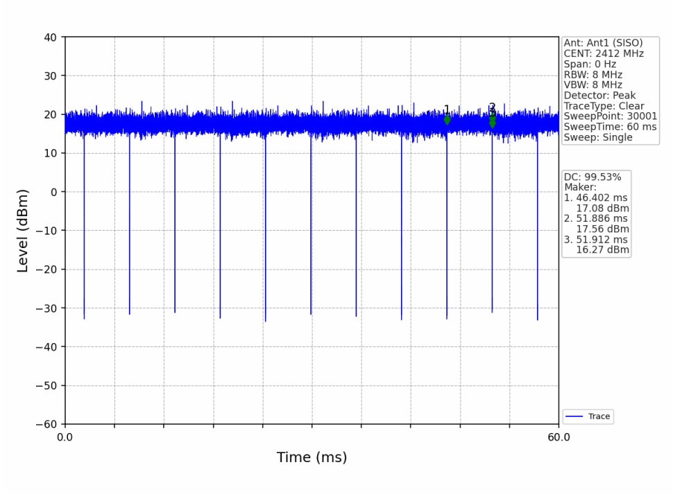
802.11g_LCH_2412MHz_Ant1 (SISO)_NTNV
