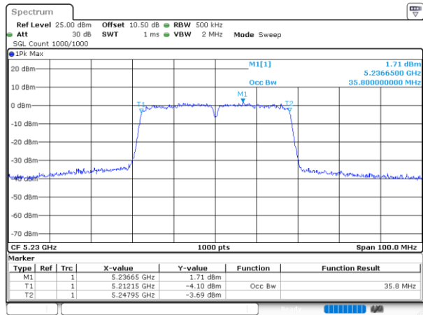
802.11n40_5230MHz
