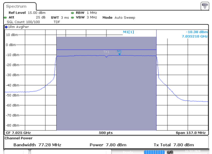
MIMO B-802.11ax-80MHz-Ch215-7025MHz-HE0
