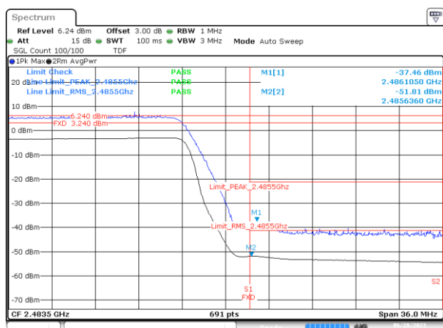
BE-R-HIGH, MIMO-A, 802.11n40-HT8, Ch11
