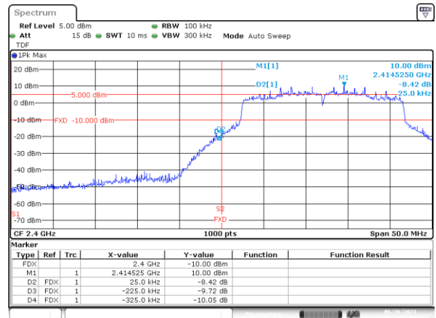
BE-NR, SISO-A, 802.11ax/be20-MCS0, Ch1
