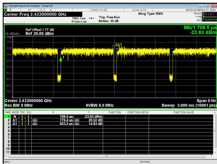
802.11n40
