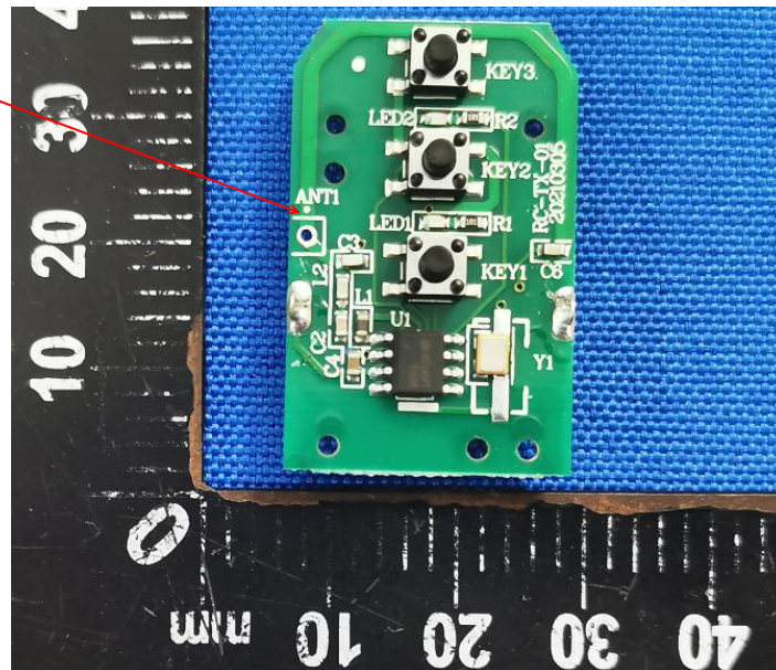
Antenna
