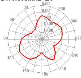
2470.000MHz E1
