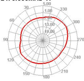
2470.000MHz H
