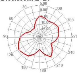
2480.000MHz E1
