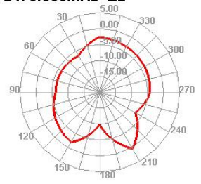
2470.000MHz E2
