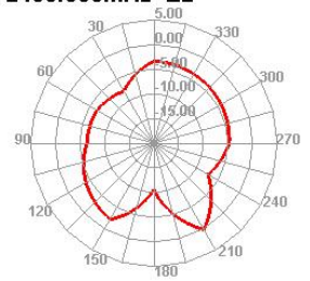
2480.000MHz E2
