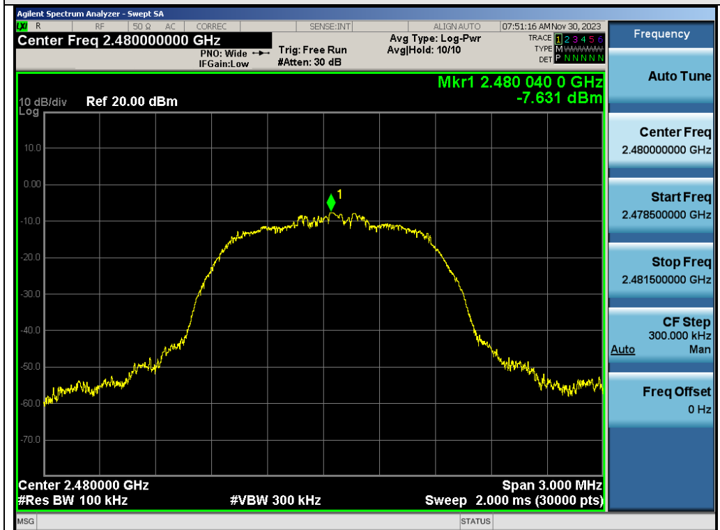
Test_Graph_EDR_ANT1_2480_2Mbps_Reference Level
