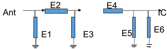
匹配电路图
