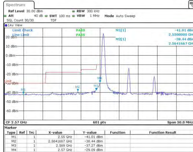
Band38-15MHz-QPSK-37825-1RB#74
