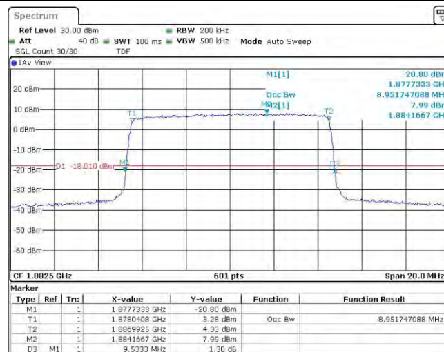
Band25-10MHz-16QAM-26365-50RB#0
