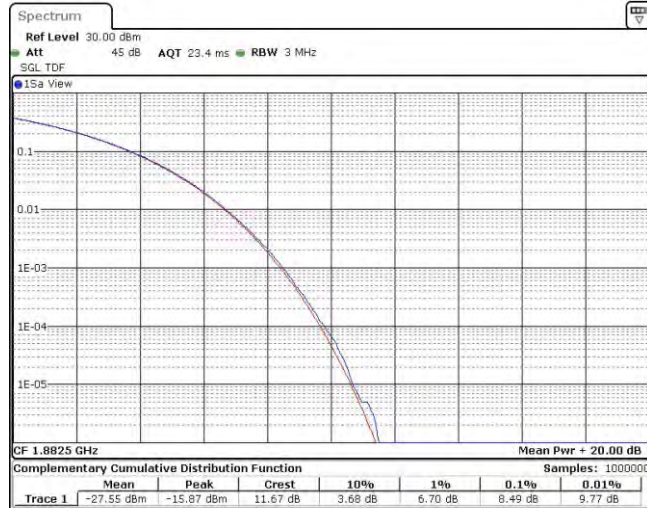
Band25-10MHz-16QAM-26365-50RB#0
