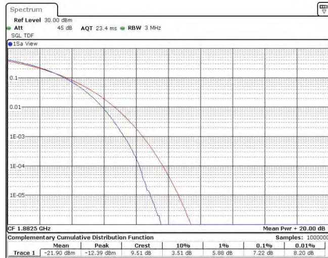
Band25-10MHz-QPSK-26640-1RB#0
