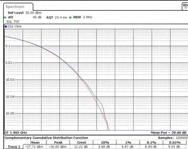
Band25-20MHz-QPSK-26590-100RB#0
