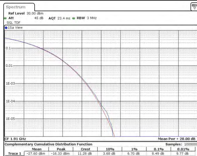
Band25-10MHz-QPSK-26640-50RB#0
