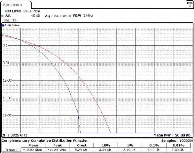
Band25-1.4MHz-QPSK-26365-6RB#0
