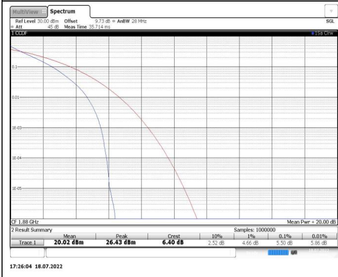
Band2-20MHz-QPSK-18900-100RB#0
