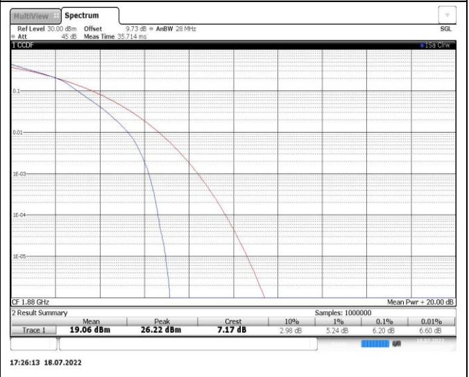
Band2-20MHz-16QAM-18900-100RB#0
