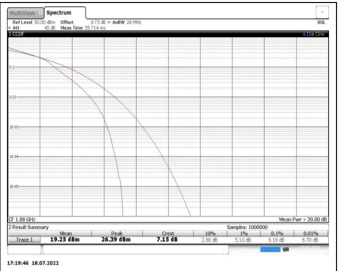
Band2-10MHz-16QAM-18900-50RB#0
