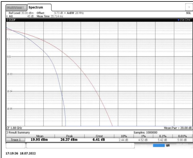
Band2-10MHz-QPSK-18900-50RB#0
