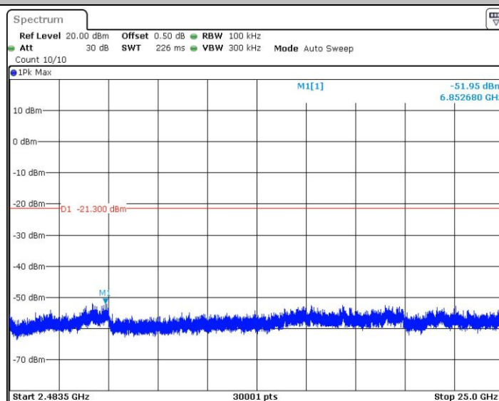
11N20SISO_Ant1_2462_2483.5~25000
