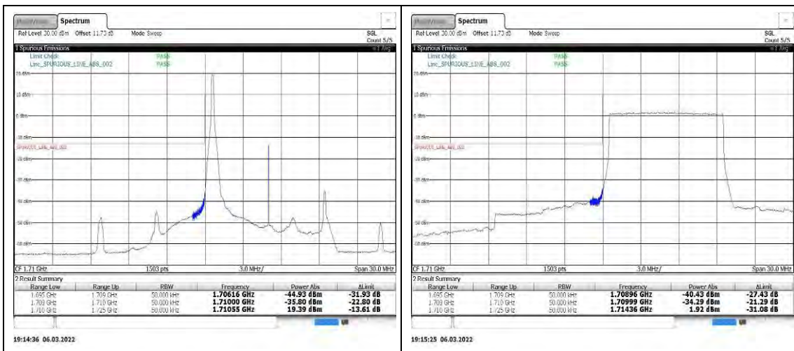
Band4-10MHz-QPSK-20000-1RB#0
