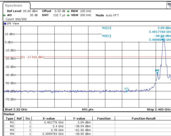
BLE_Low_2402
