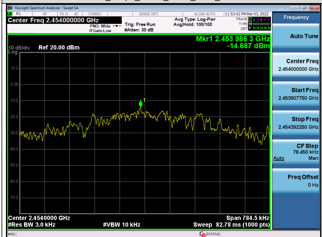
Test_Graph_GFSK_ANT1_2454_PSD
