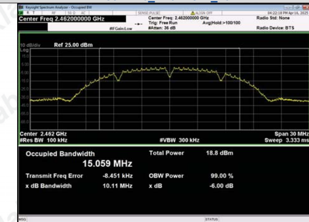
IEEE 802.11b_Channel 11_20MHz
