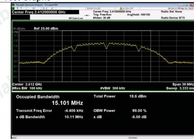
IEEE 802.11b_Channel 1_20MHz
