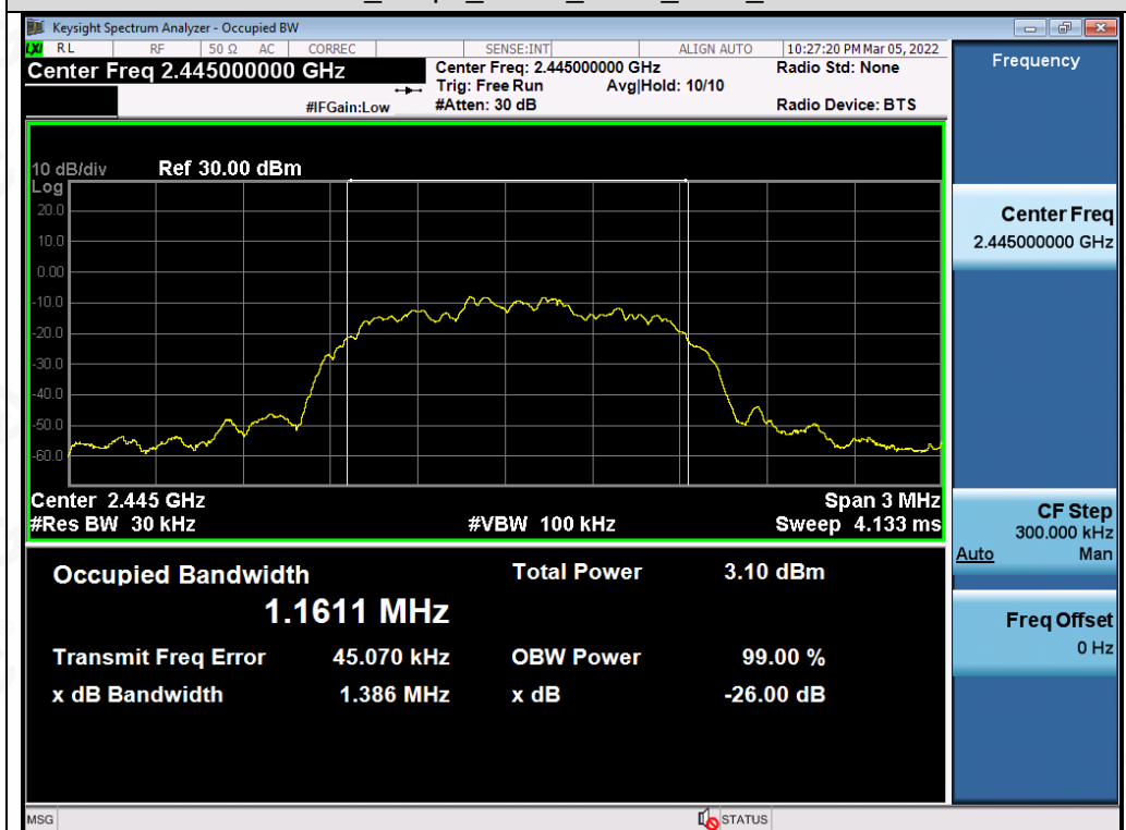
Test_Graph_GFSK_ANT1_2445_OBW
