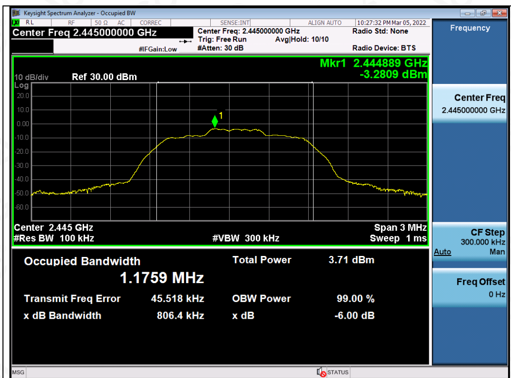
Test_Graph_GFSK_ANT1_2445_DTSBW
