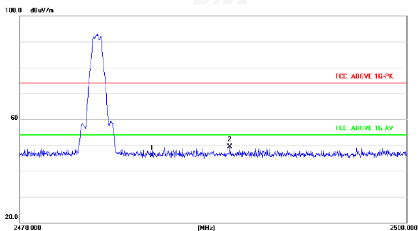
2482.5MHz Horizontal
