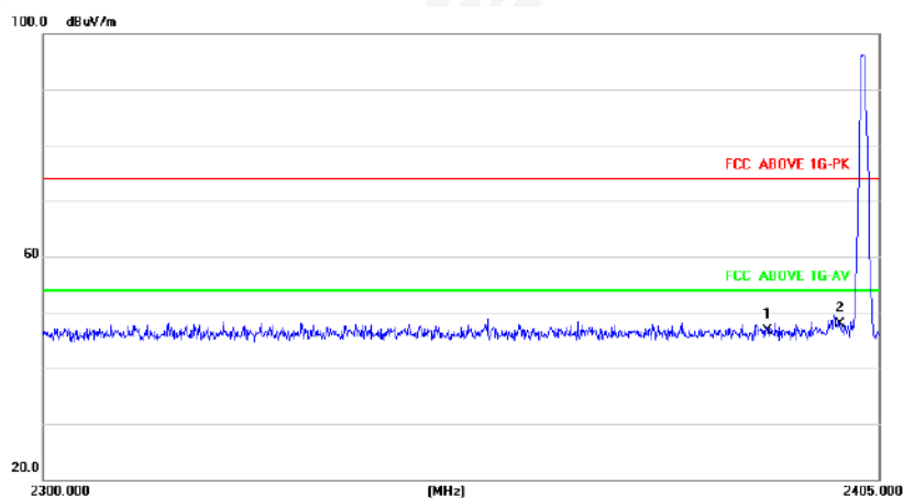
2401.25MHz Horizontal
