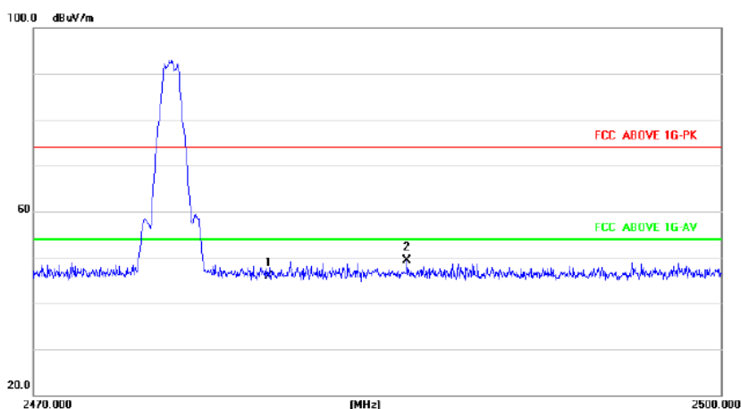
2482.5MHz Vertical
