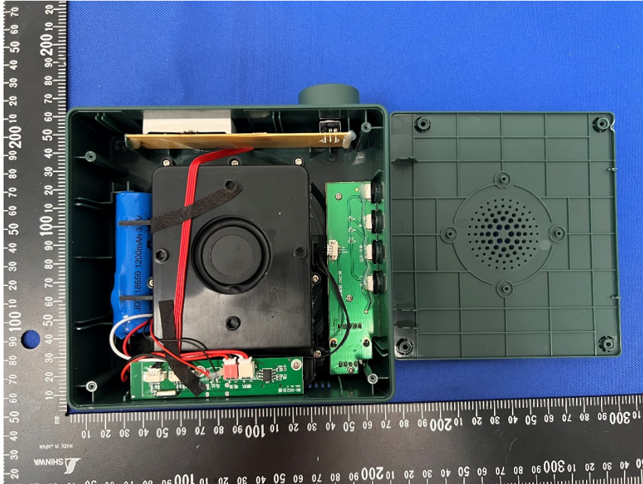
PCB ANT
