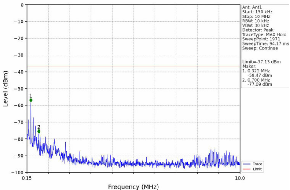
2.4g_HCH_2479MHz_Ant1_NTNV
